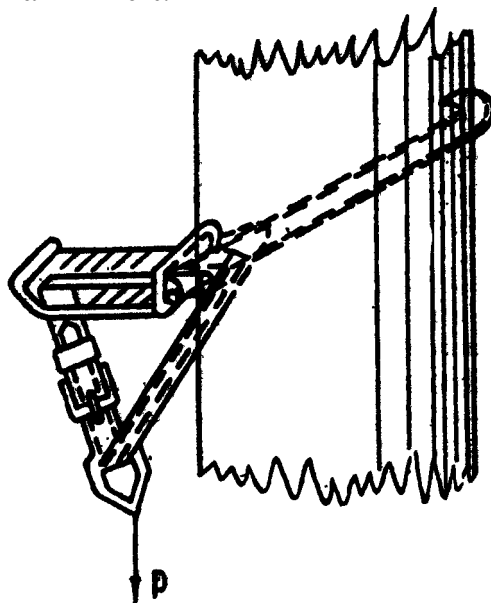
Рис. 6.1. Схема испытания монтерских когтей (P — испытательная нагрузка)
