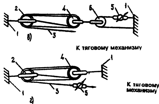
Рис. 4.4. Схема испытания многорольных блоков и полиспастов:
