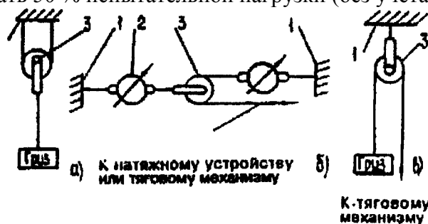
Рис. 4.3. Схема однорольных блоков:
