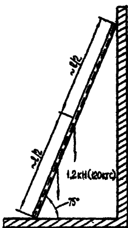
Рис. 5.5. Схема испытания приставной лестницы
