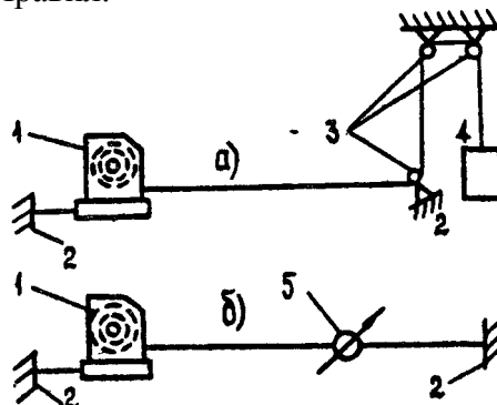
Рис. 4.1. Схемы испытания лебедок:
