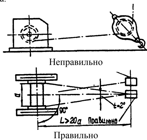
Рис. 4.2. Намотка каната на барабан лебедки
